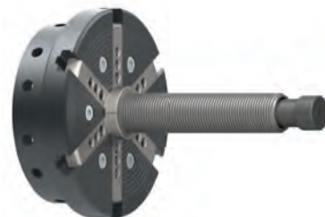
QuickHub в закрытом состоянии, минимальный диаметр центрального отверстия диска 53,5 мм (без дополнительных насадок).
