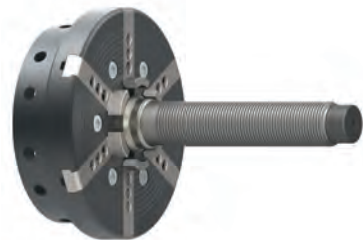
QuickHub в раскрытом состоянии, максимальный диаметр центрального отверстия диска 77,1 мм (без дополнительных насадок).
